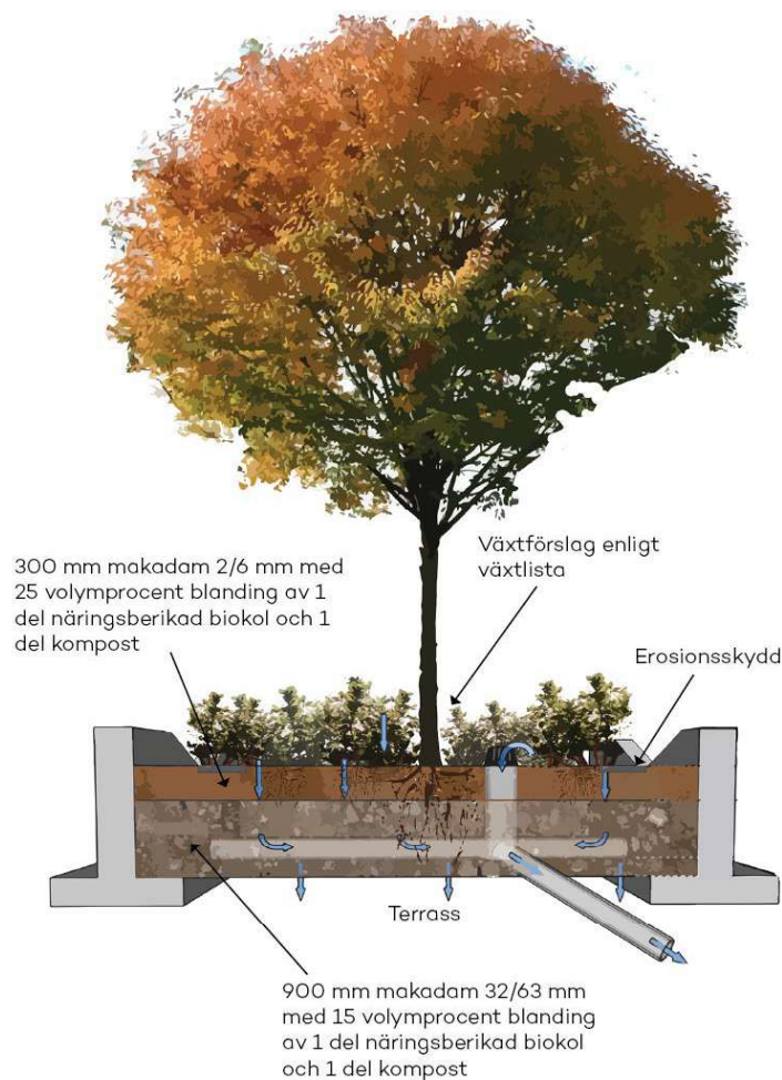
Figur 16. Typsektion för skelettjord med biokol. Den föreslagna dagvattenlösningen ska inrymma plantering av enkelsidig trädallé och mindre vegetation såsom exempelvis buskar. Skelettjord bidrar
